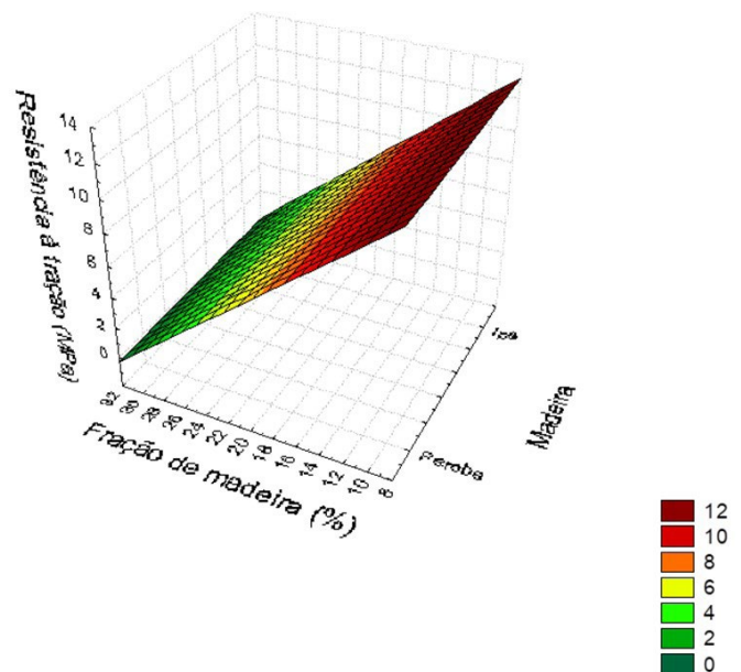
Figura 1 – Superfície de resposta mostrando a influência do tipo de reforço e da fração volumétrica de reforço sobre a resistência à tração dos compósitos
