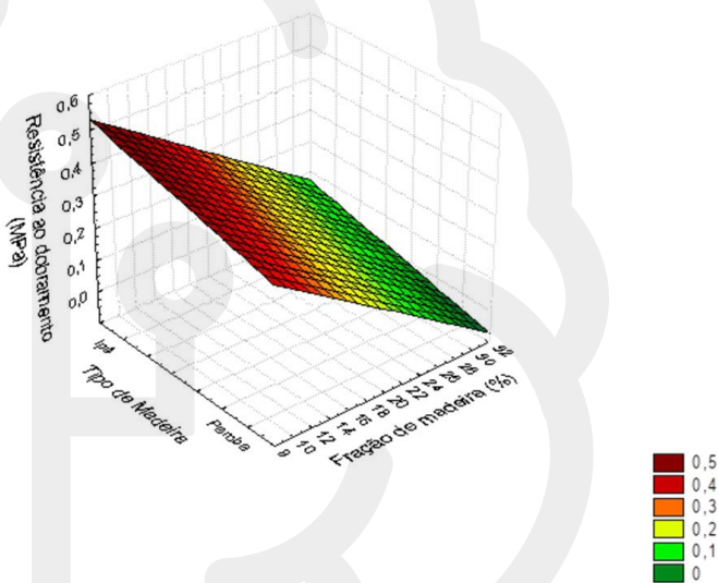
Figura 2 – Superfície de resposta mostrando a influência do tipo de reforço e da fração volumétrica de reforço sobre a resistência à ruptura por flexão dos compósitos
